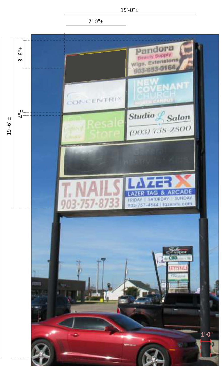
EXISTING SCALE: 3/16" = 1' - 0"
